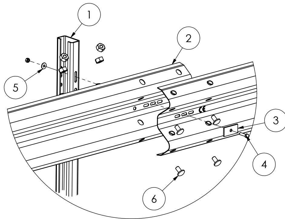
DÉTAIL A ECHELLE 1 : 10
