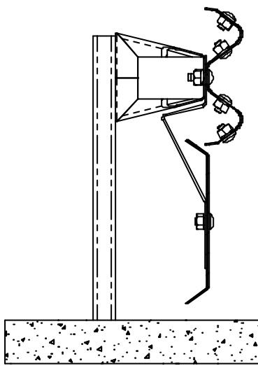
Détail montage bras type L
